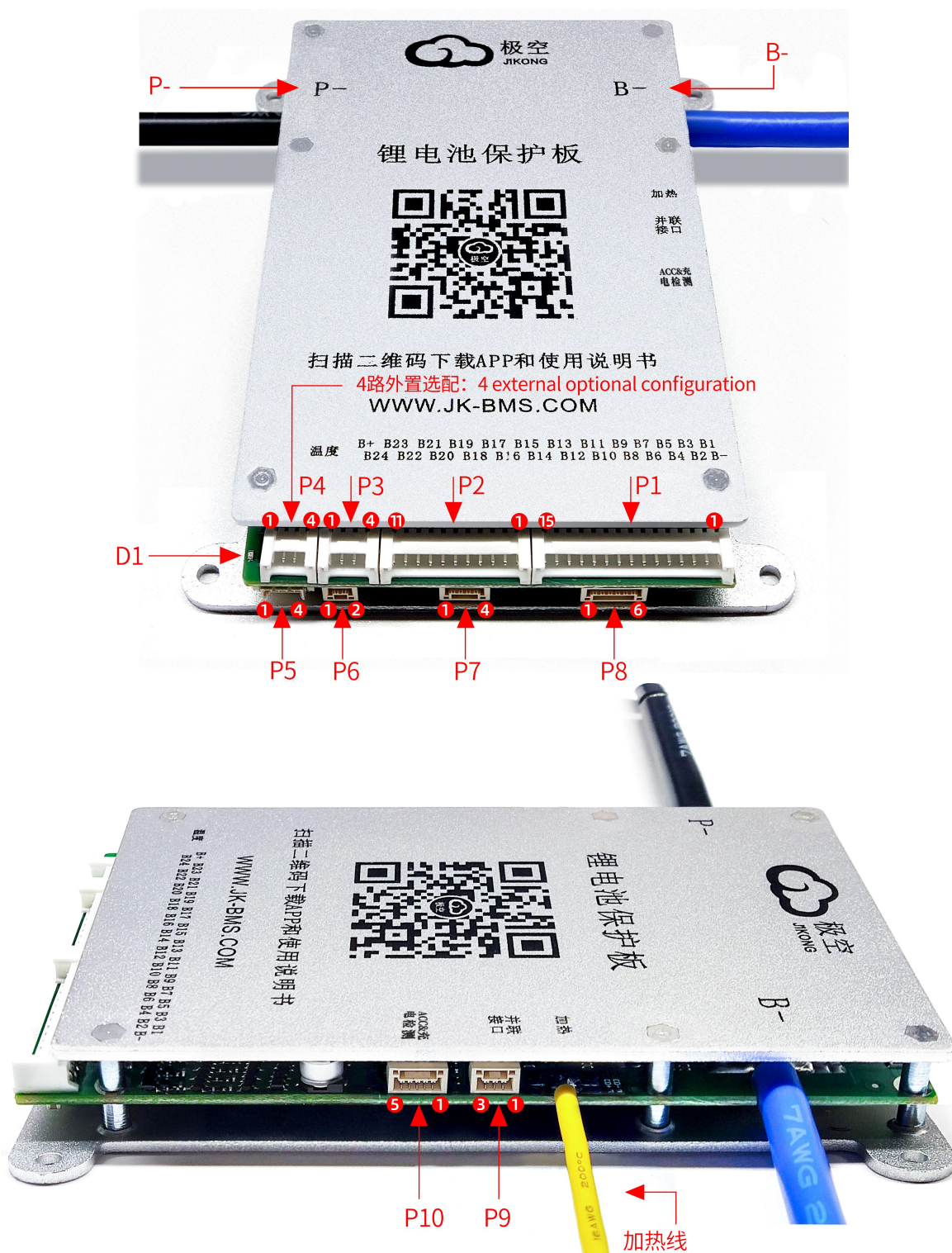
JK-BD6AxxS-6P/8P连接器示意图
