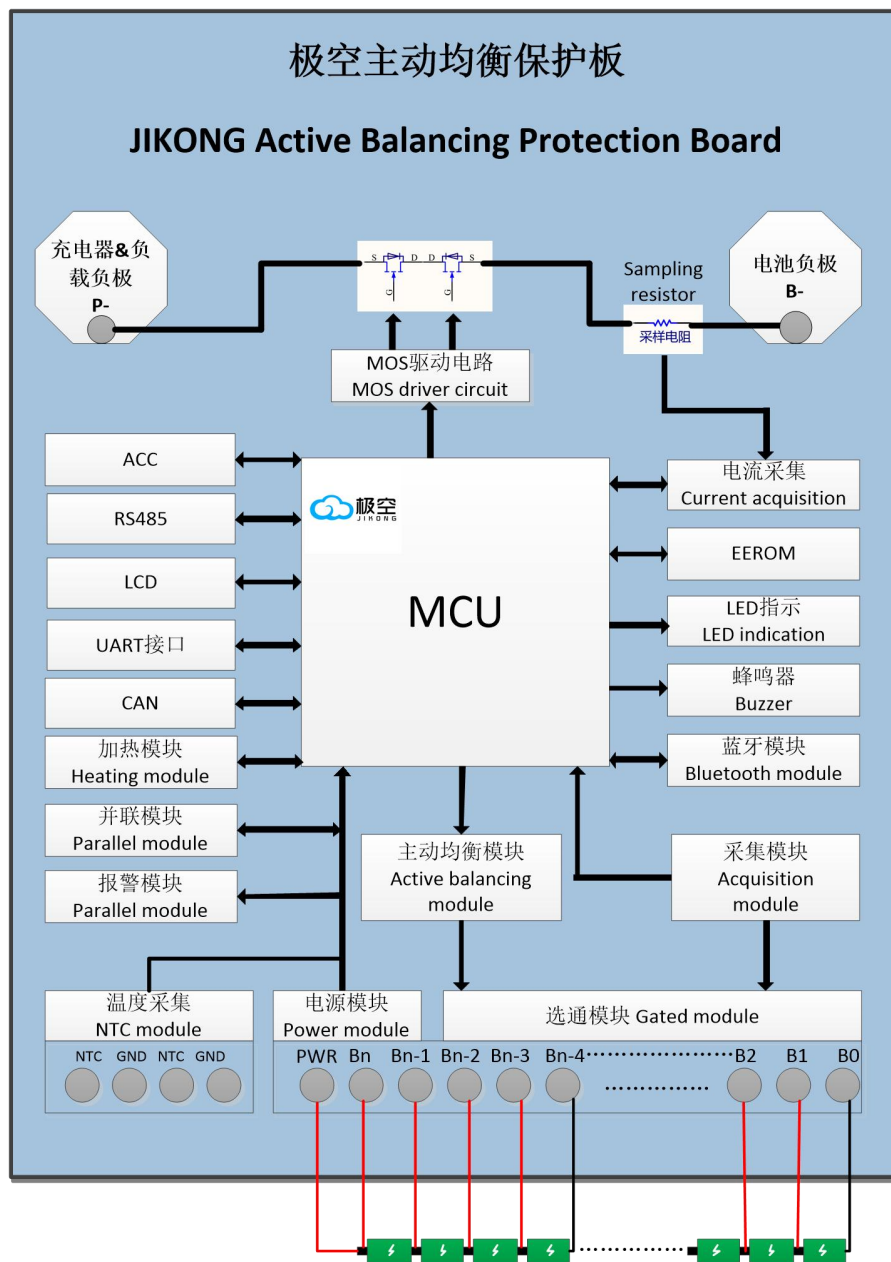
JK-BD6AxxS-6P/8P结构框图
